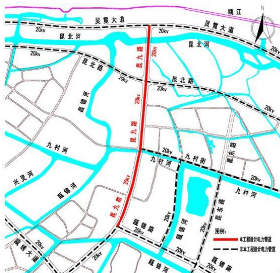
图 1-15 电力排管系统图
