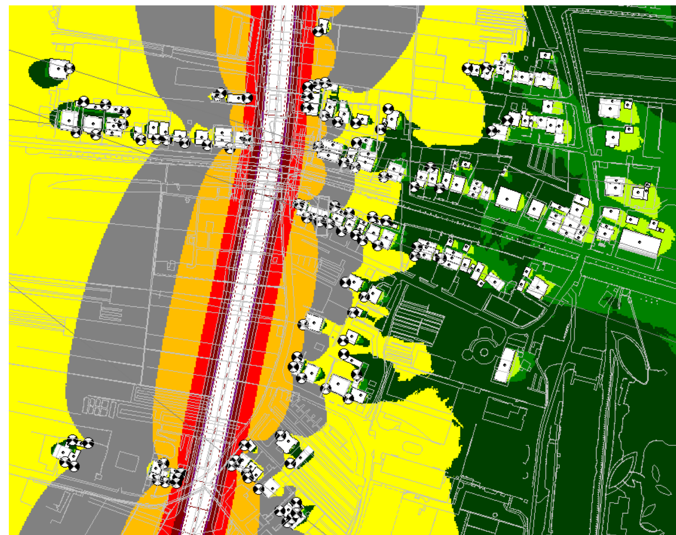
九村村远期敏感点夜间等声级线图
