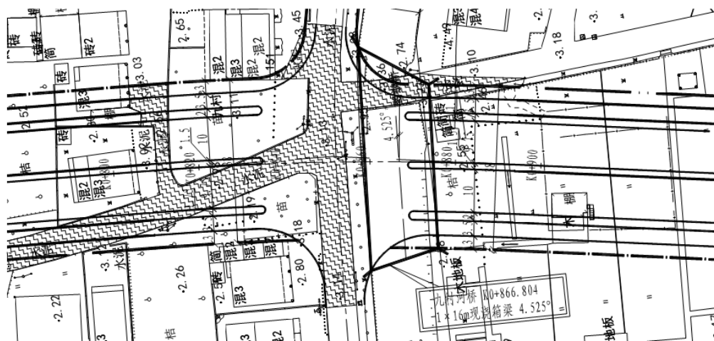
图 1-8 九村河桥平面图
