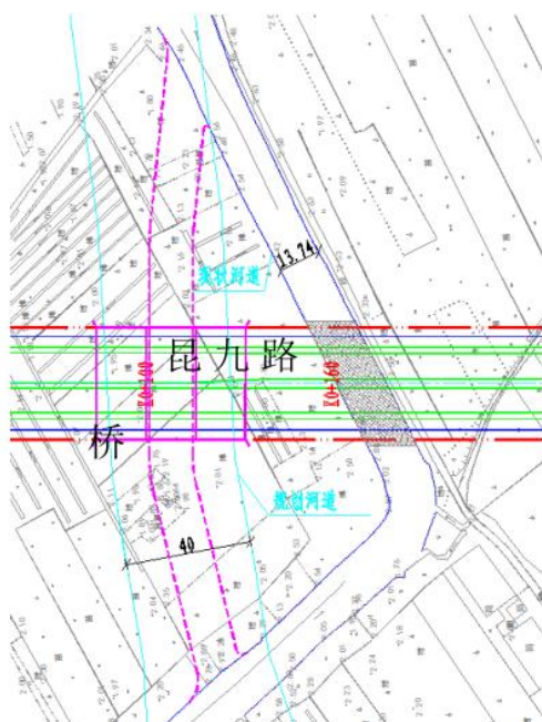
河道改移方案图
