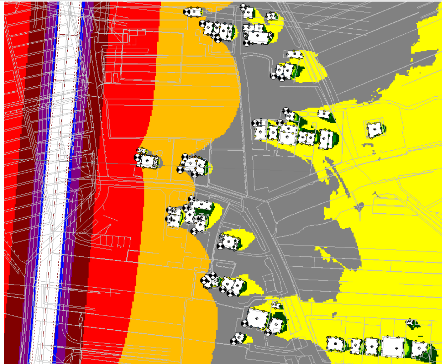
北段村远期敏感点昼间等声级线图
