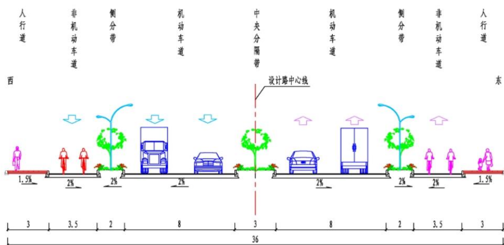
图 1-4 道路标准横断面图
