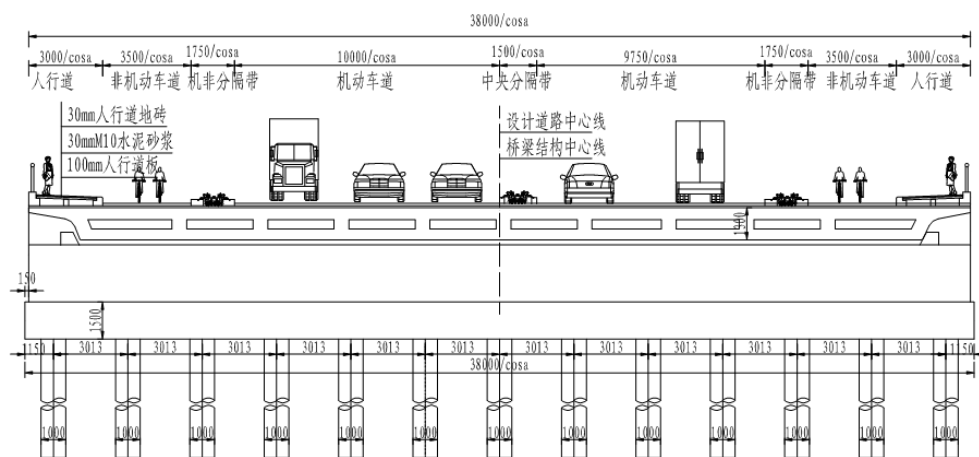
图 1-10 九村河桥标准断面图
