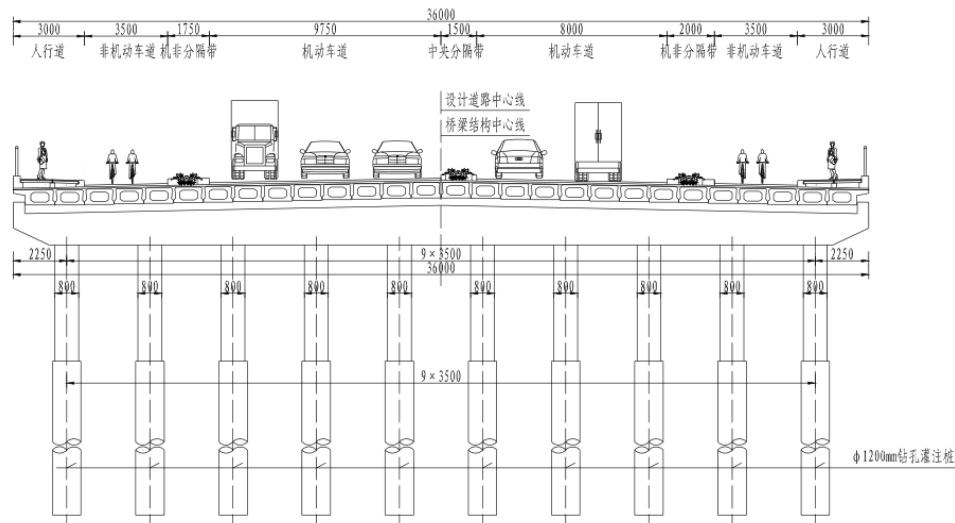
图 1-7 昆九路桥标准断面图
