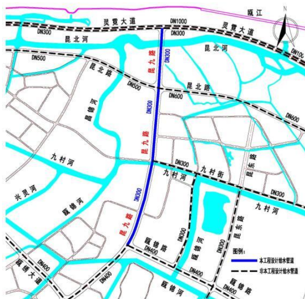
图 1-14 给水管道系统图
