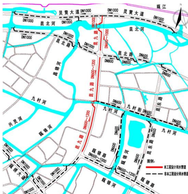
图 1-12 雨水管道系统图
