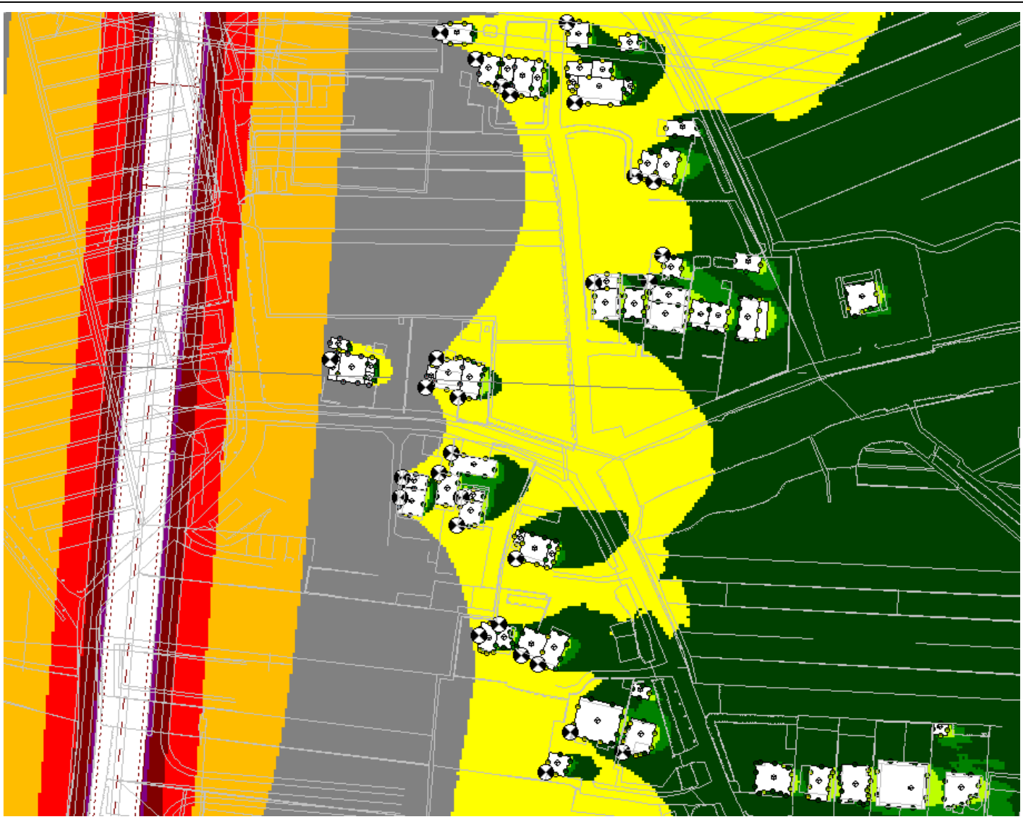
北段村远期敏感点夜间等声级线图
