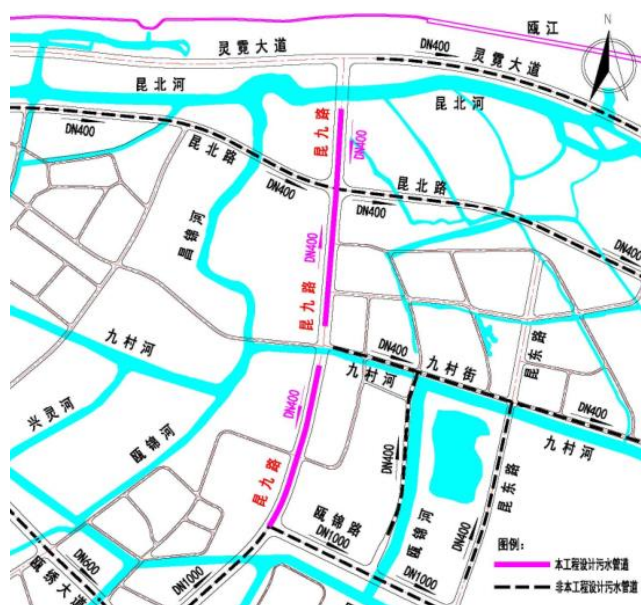
图 1-13 污水管道系统图
