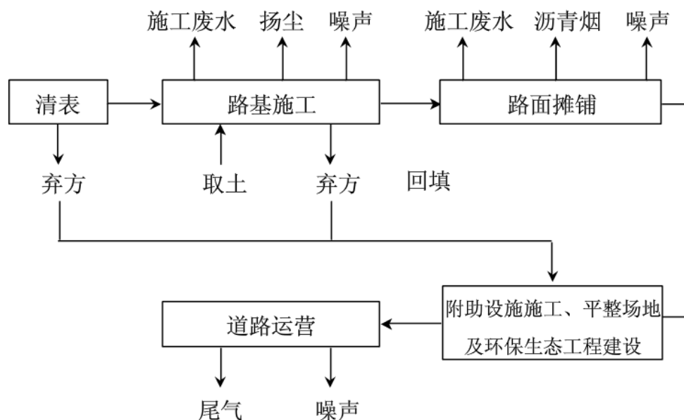
图 5-1 施工期、营运期产污工艺流程图
