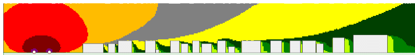
九村村远期敏感点夜间立面预测图
