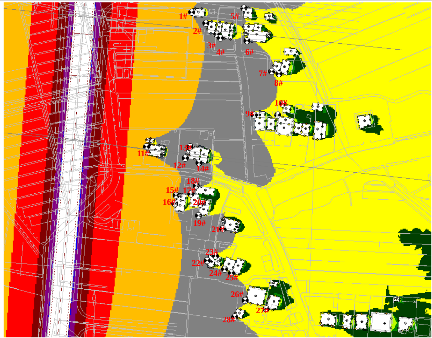
北段村近期敏感点昼间等声级线图
