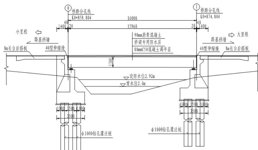
图 1-9 九村河桥立面图
