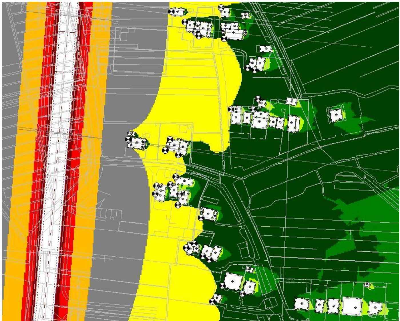
北段村近期敏感点夜间等声级线图
