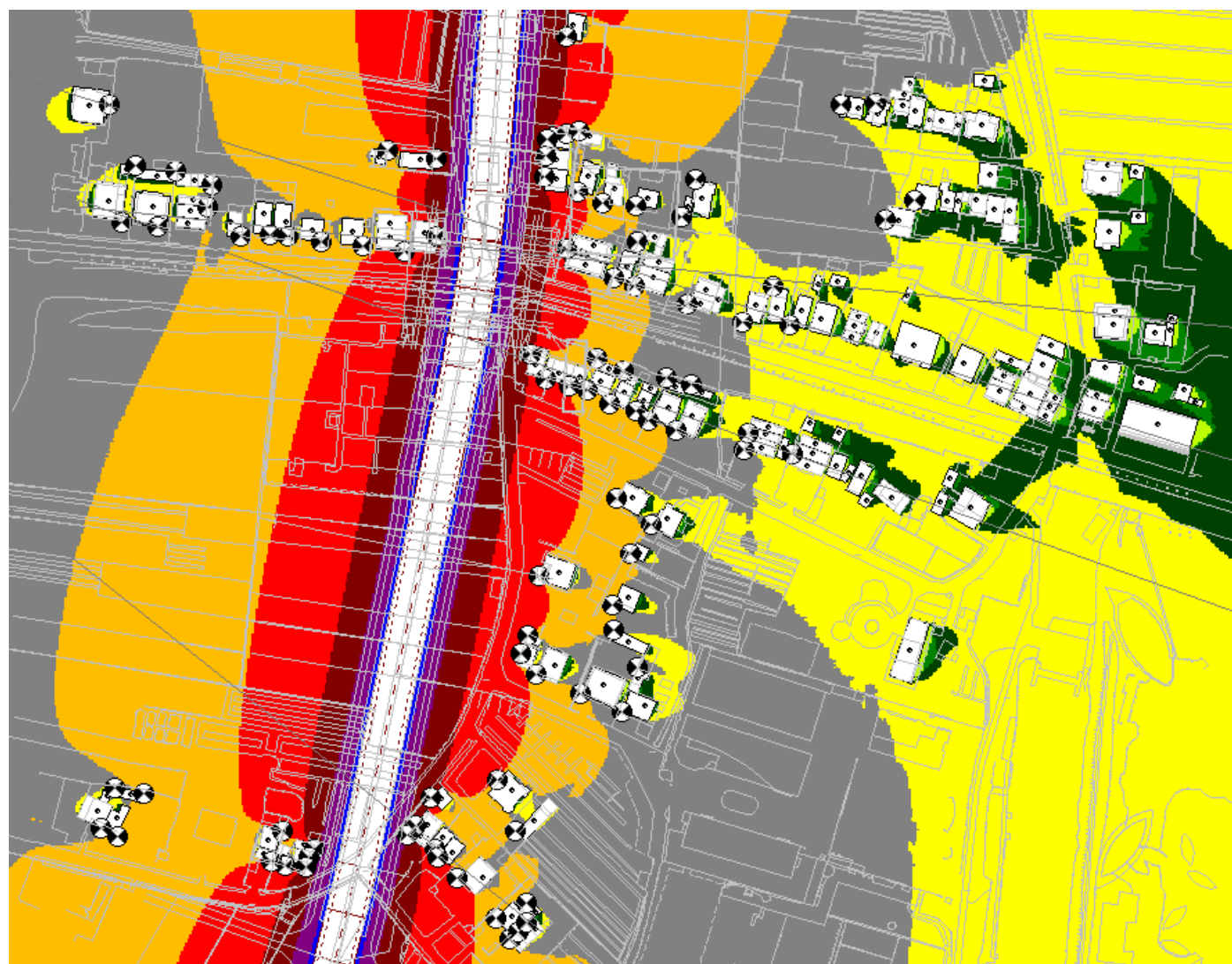
九村村远期敏感点昼间等声级线图
