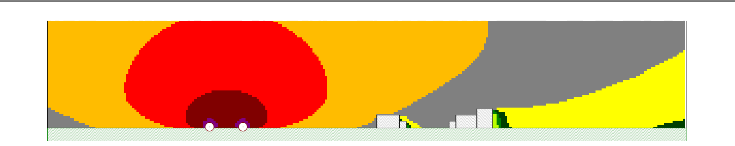
北段村远期敏感点夜间立面预测图
